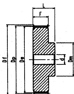
H 100 - pro řemen širé 1" (25.40 mm)
