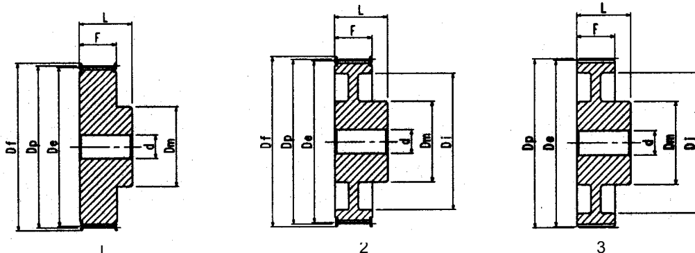
H 200 - pro řemen širé 2" (50.80 mm)
