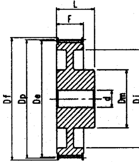
H 300 - pro řemen širě 3" (76.20 mm)
