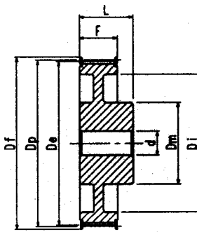
H 150 - pro řemen širě 1"1/2 (38.10 mm)
