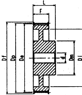
H 100 - pro řemen širé 1" (25.40 mm)
