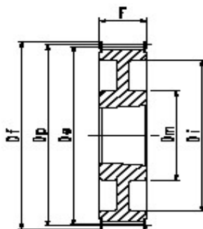
H 100 - pro řemen širě 1" (25.40 mm)
