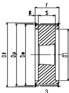
H 300 - pro řemen širě 3" (76.20 mm)
