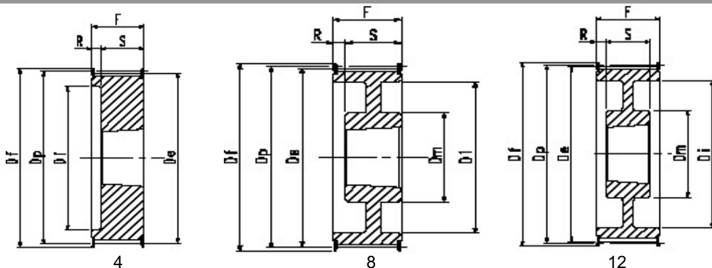
H 100 - pro řemen širě 1" (25.40 mm)
