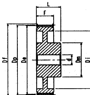
H 075 - pro řemen širě 3/4" (19.05 mm)
