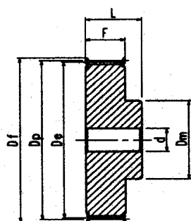
H 075 - pro řemen širě 3/4" (19.05 mm)
