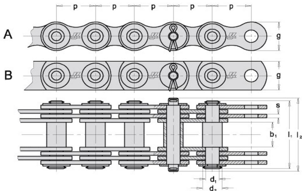
Gallové řetězy s podložkami (DIN 8150)
