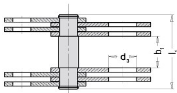
Závěsné články nerozebiratelné
