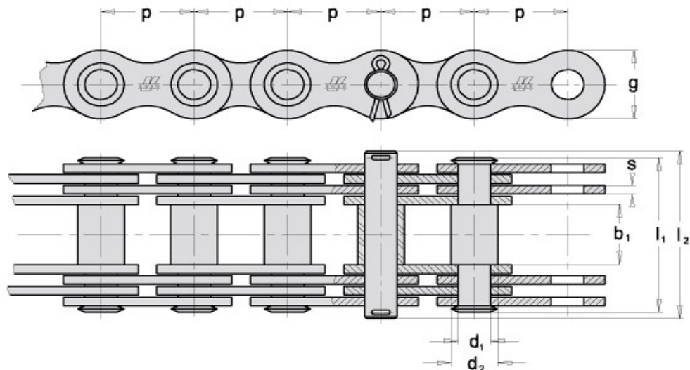
Gallovy řetězy bez podložek (DIN 8150)
