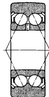
Řada 3058/00/C-ZZ
