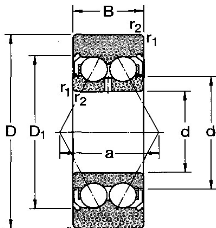
Řada 3057/00/C-ZZ
